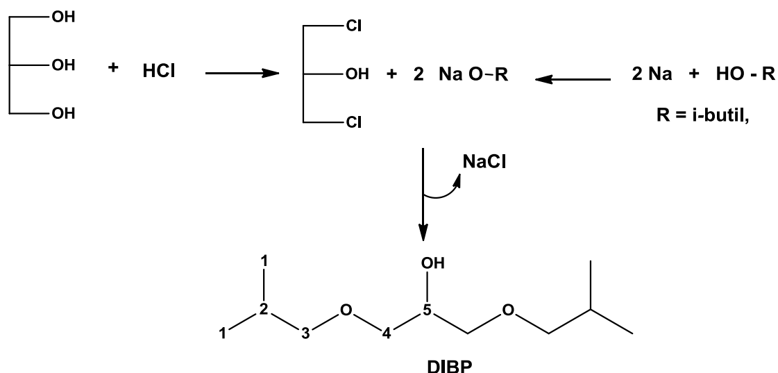
Figura 1: Esquema para a obtenção do biocombustível de segunda geração.
