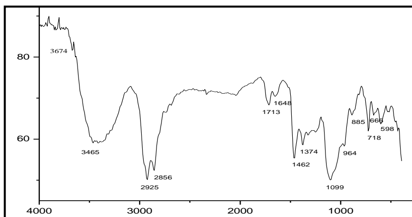
Figura 3 - Espectro de IV do 1,3-diisobutóxiopropan-2-ol (DIBP) em KBr \text{cm}^{-1}
