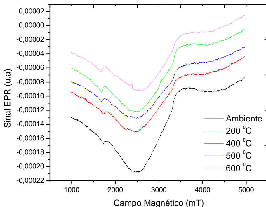
Figura 3. Espectros de RPE de fragmento de cerâmica encontrado no sítio Justino.
