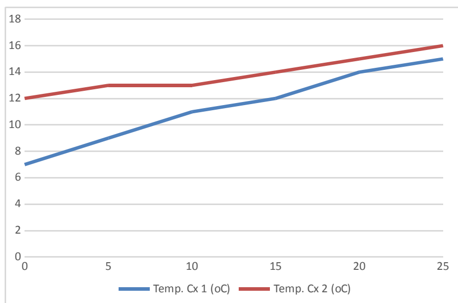
Figura 7. Temperaturas da Caixa 1 (bomba de calor geotérmico) e Caixa 2. Fonte: próprio autor
