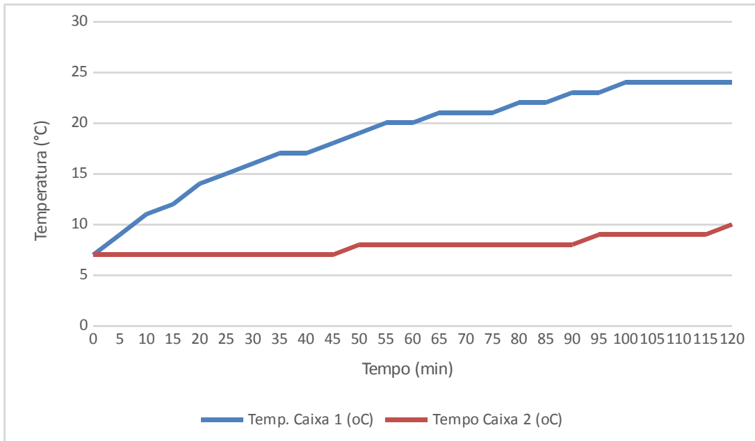
Figura 5. Temperaturas da Caixa 1 (bomba de calor geotérmico) e Caixa 2. Fonte: próprio autor
