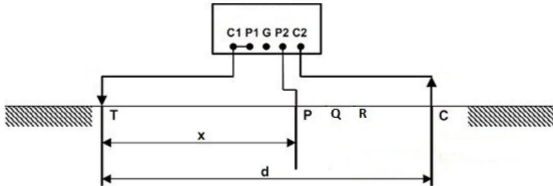
Figura 1 – Medição da resistência de aterramento. Fonte: elaborado pelo autor.
