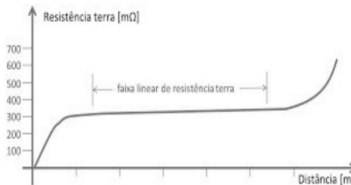
Figura 2 – Curva característica da resistência de aterramento. Fonte: Paulino, 2012.
